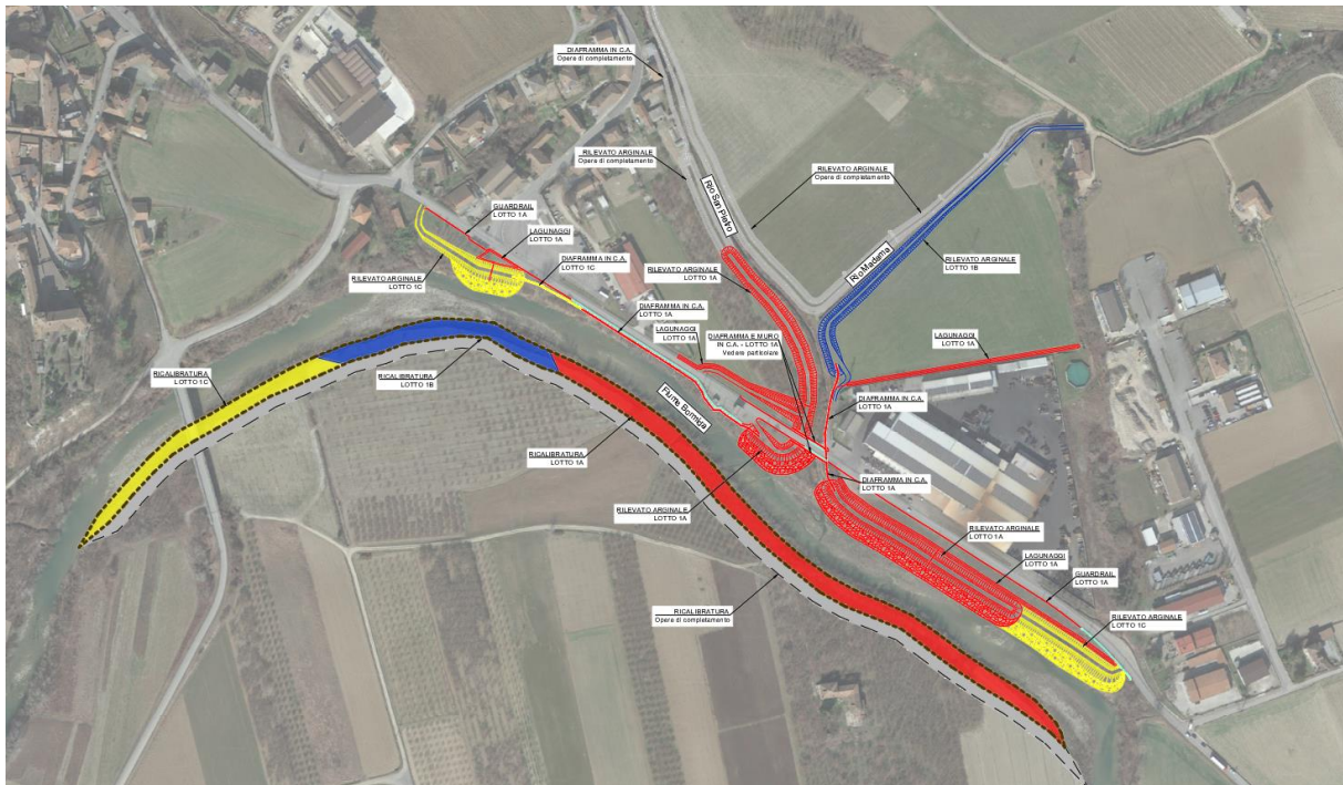
Figura 3.1: Planimetria di progetto
