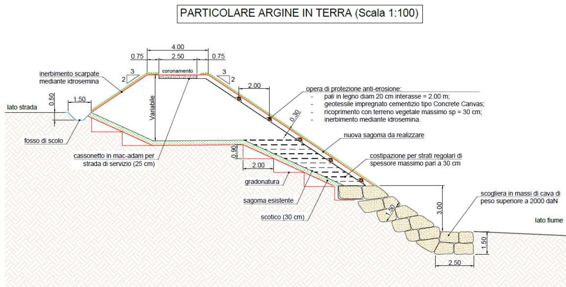
Figura 3.2: Particolare argine in terra progetto generale
