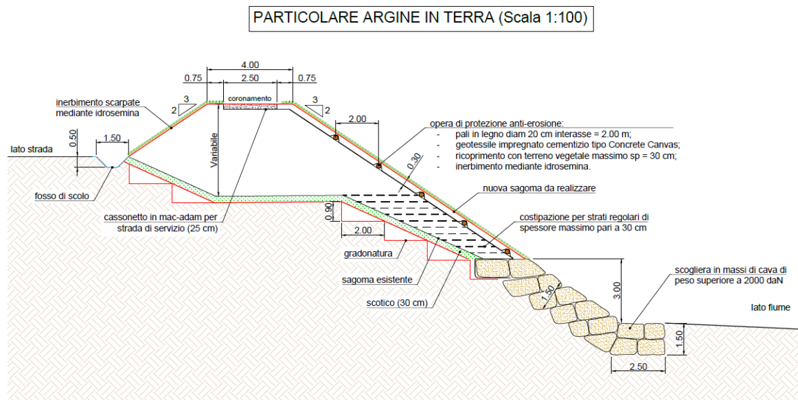
Figura 3.2: Particolare argine in terra previsto nel progetto generale
