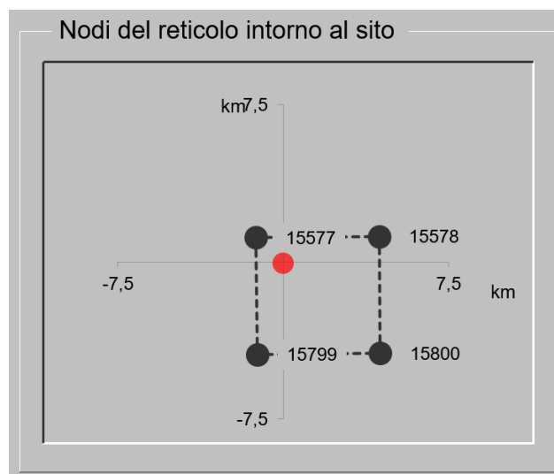
Figura 14 – Nodi del reticolo NTC08 attorno al sito
