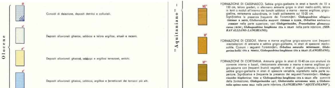
Figura 2 - Estratto Carta Geologica d'Italia alla scala 1:100000 – Fogli n° 69 – Asti e n° 81 Ceva
