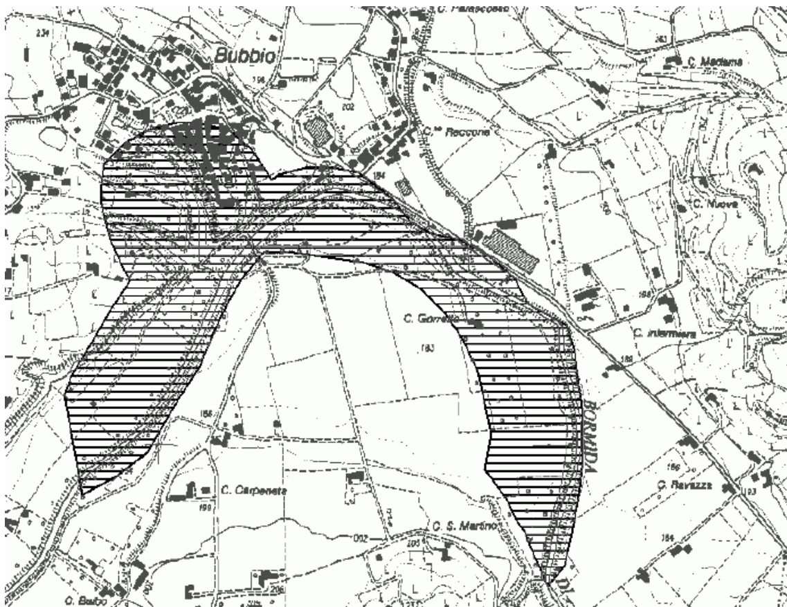
Figura 6.1: Estratto carta della pericolosità da alluvione del P.G.R.A: Pericolosità MOLTO ELEVATA
